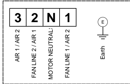
Twinflow Fan Terminal Box
