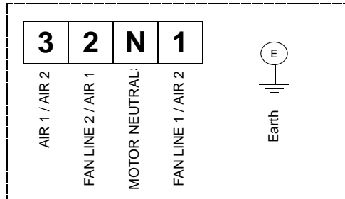
Twinflow Fan Terminal Box
